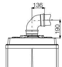
Doppelrohr-System horizontal \varnothing 80/125
