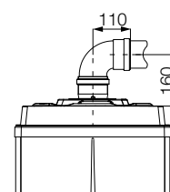
Abgas-System horizontal \varnothing 80
