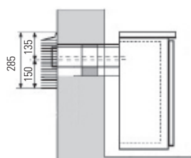
Ausführung Fassadengitter
