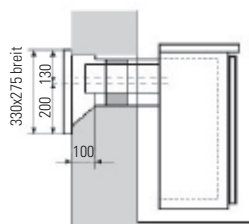
Ausführung Mauerkasten
