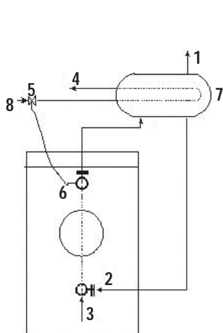
Hydraulikschema
